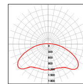
60W-5000K-160°
