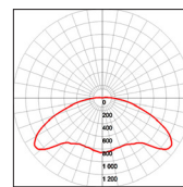
40W-5000K-160°
