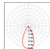
200W-5000K-50°
