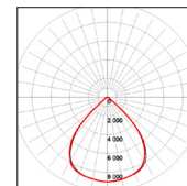
100W-5000K-90°
