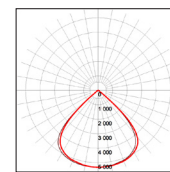
60W-5000K-90°
