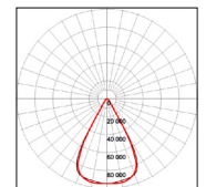
600W-5000K-60°
