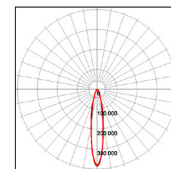
600W-5000K-20°
