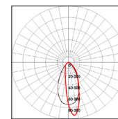
600W-5000K-30x55°
