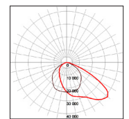
600W-5000K-60x110°
