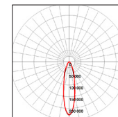
600W-5000K-30°
